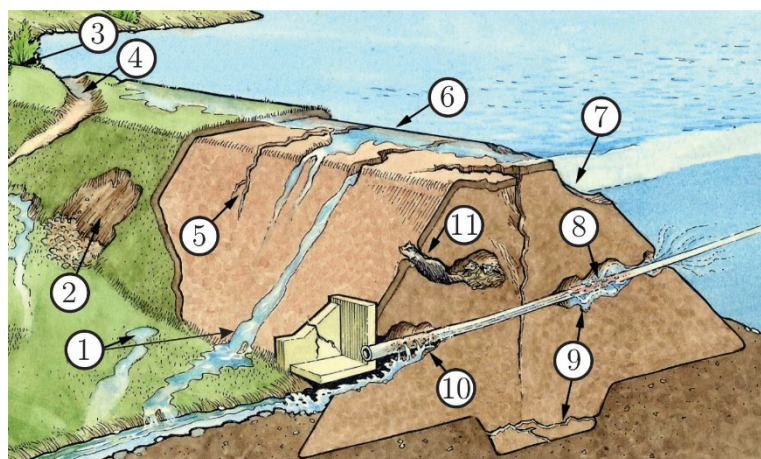
слика 1. Узроци оштећења насипа: 1 – процуривање; 2 – одроњавање; 3 – корење запуштеног растиња; 4 – „дивље“ стазе; 5 – пукотине изазване оптерећењем тла; 6 – слегање круне услед прекомерног саобраћаја (може довести до преливања насипа); 7 – дејство таласа; 8 – ерозија тла око цеви побијеном кроз тело насипа; 9 – унутрашња ерозија; 10 – испирање тла услед цурења из оштећене цеви; 11 – кртичњаци (према “ASDSO Lessons Learned”, damfailures@damsafety.org )
